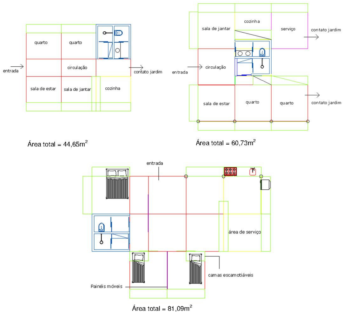
FIGURA 7- Plantas esquemáticas de arranjo dos módulos do sistema habitacional: 44,65 m 2 para famílias menores, pessoas vivendo sós, casais sem filhos. 60,73 m 2 para familiar nucleares sem expansão e 81,09 m 2 para familiar nucleares com expansão.
