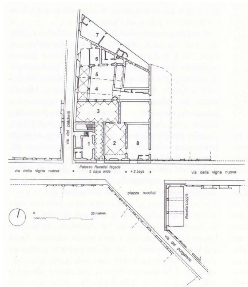
Figura 27 – Planta baixa do pavimento térreo do Palazzo Rucellai, onde os números indicam a posição das oito edificações originais que formaram o palácio. Fonte: TAVERNOR, 1998, p. 82.
