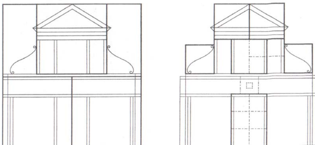
Figuras 25 e 26 Estudo das proporções na fachada de S. M. Novella proposto por Rudolf Wittkower. Fonte: WITTKOWER, 1995, p. 69.
