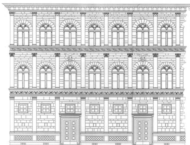
Figura 36 Fachada do Palazzo Rucellai, reconstituída pelo Alberti Group. Fonte: TAVERNOR, 1998, p. 87.
