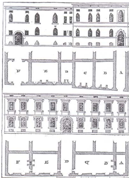
Figura 28 – Proposição para a unificação e modernização da fachada de duas residências segundo Sebastiano Serlio. Fonte: SERLIO, 1978, p. 171.
